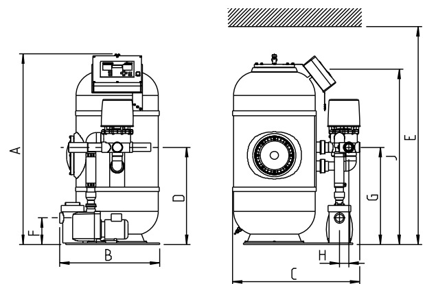
Abb. 3 Maßzeichnung Filteranlage GENO-mat® F 610 A
