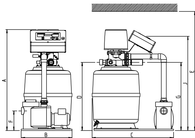
Abb. 2 Maßzeichnung Filteranlage GENO-mat® F 500 A
